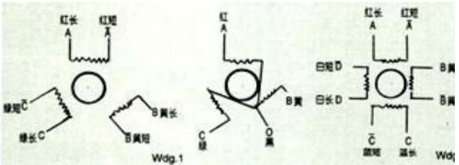
接线图1
