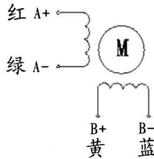
(电机线)
