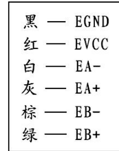
(编码器线)
