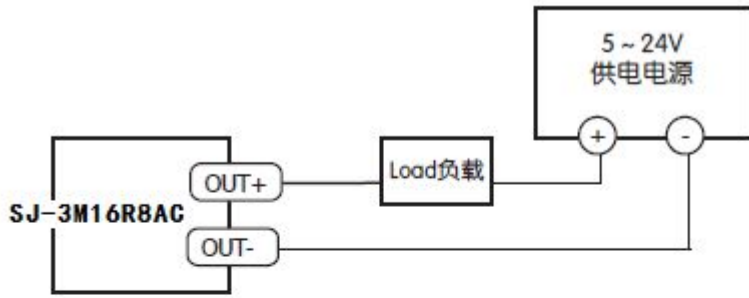
灌电流输出的连接方式
