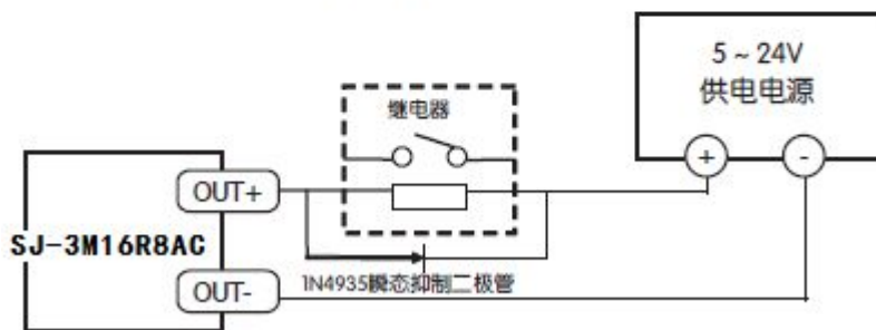
驱动一路继电器的连接方式
